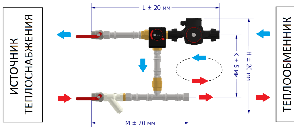
Схема смесительного узла обратной конфигурации без байпаса
